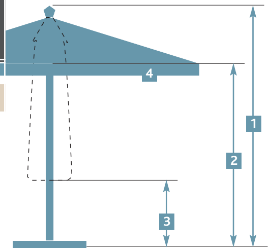
Modèle standard : toile Orchestra SANS LAMBREQUIN + GOUTIÈRE
