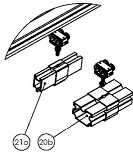
DÉTAIL A ECHELLE 1:5
