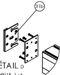
DÉTAIL C ECHELLE 1:6
