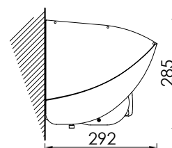
Montaggio con tettuccio Installation with a hood
