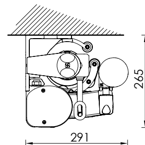
Montaggio a soffitto Ceiling installation
