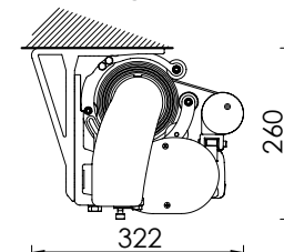
Montaggio a soffitto Ceiling installation
