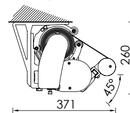
Montaggio a soffitto 45° Ceiling installation 45°
