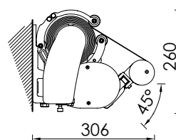
Montaggio a parete 45° Wall installation 45°
