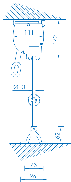
Montaggio a soffitto Ceiling installation
