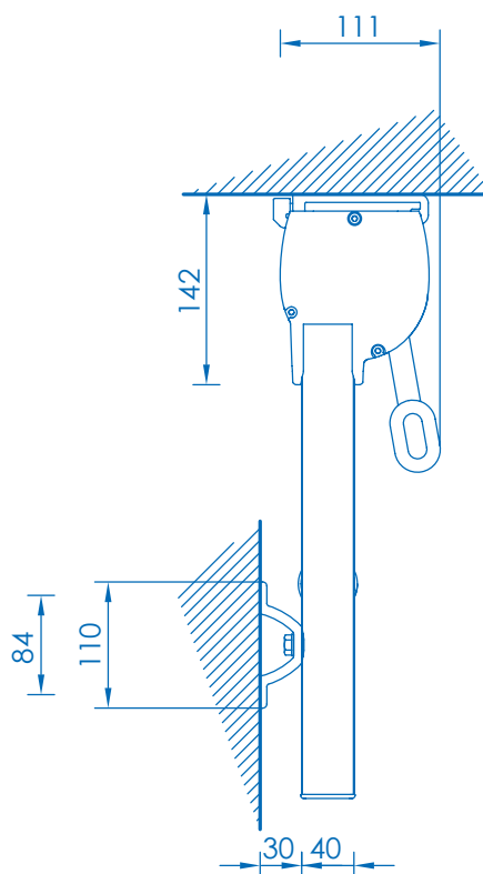
Montaggio a soffitto Ceiling installation
